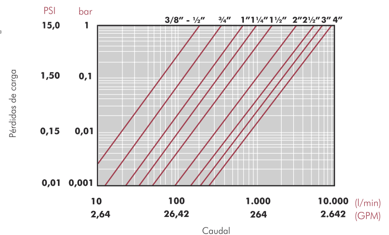
Diagrama de pérdidas de carga
